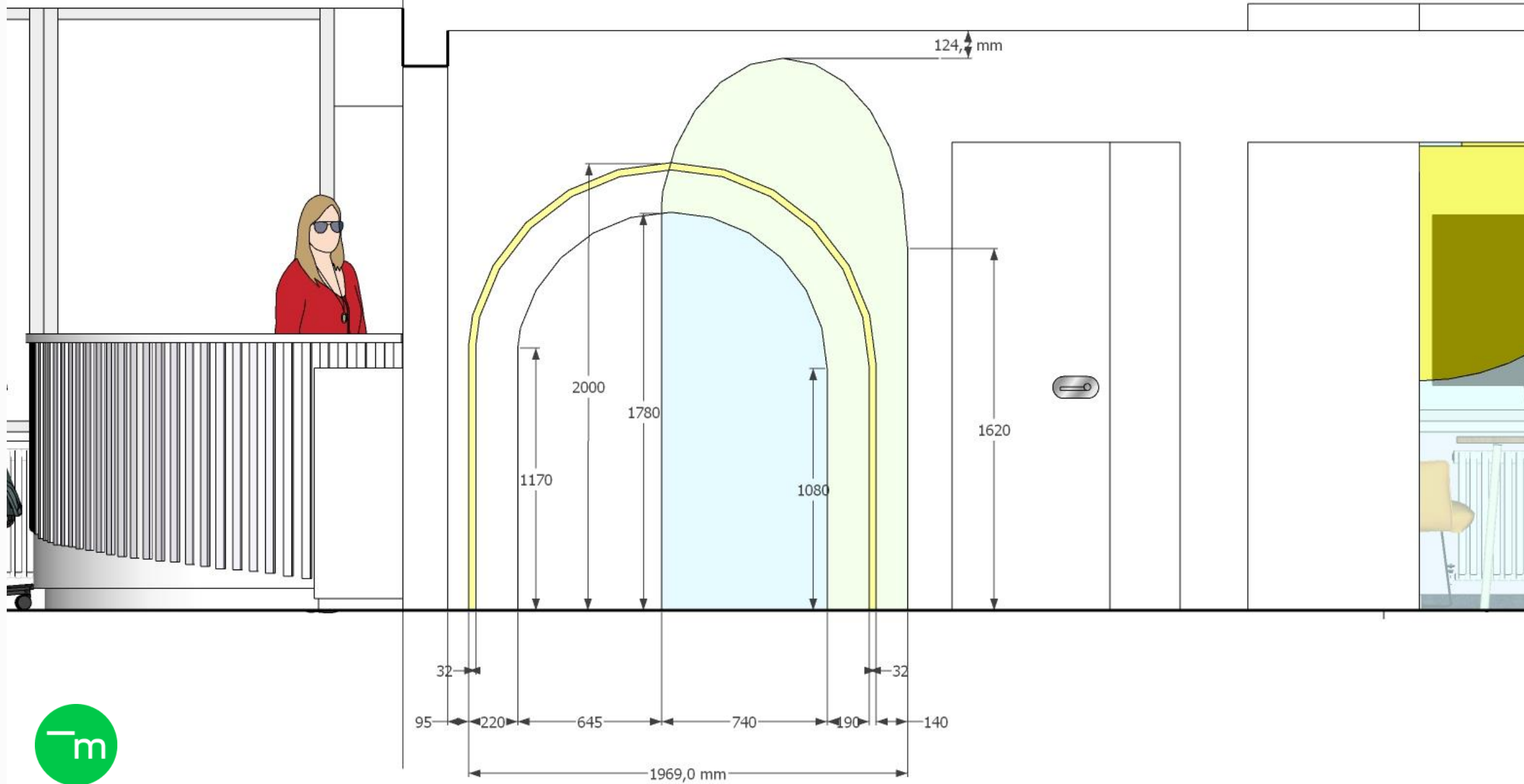
Развёртка 12.2
